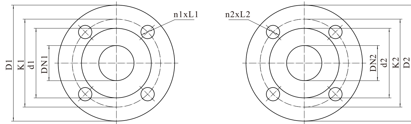
Патрубок всасывания
