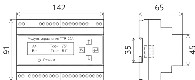
Внешний вид и габаритные размеры TTR-02A/TTR-12A
