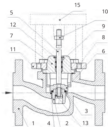
Устройство неразгруженного по давлению клапана DN 15 - DN 32
