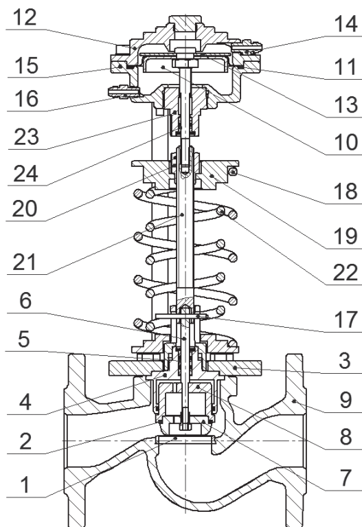
Устройство регулятора давления RDT-T
