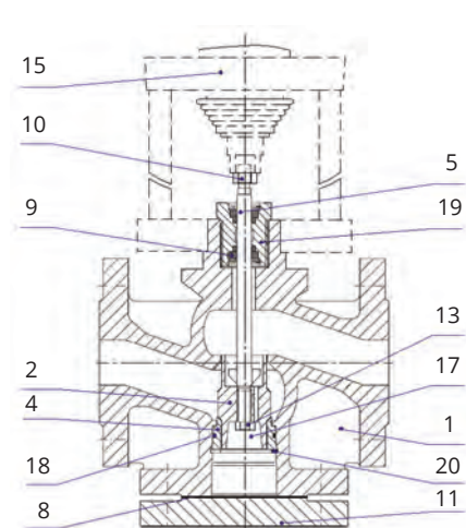
Устройство разгруженного по давлению клапана DN 65 - DN 200
