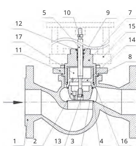
Устройство разгруженного по давлению клапана DN 40 - DN 200
