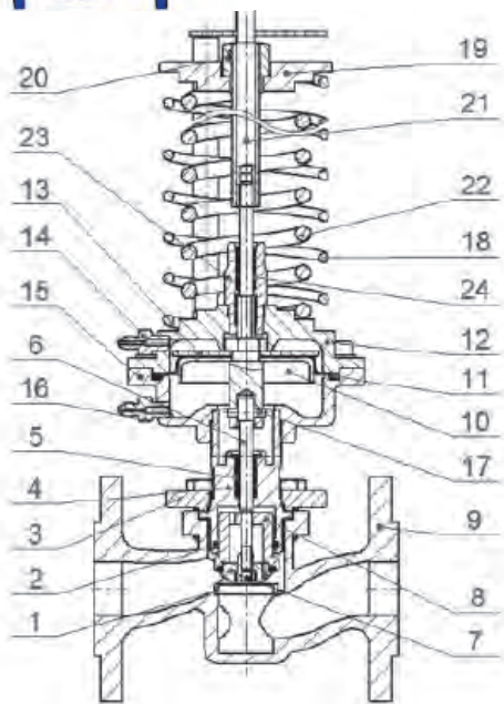
Устройство регулятора
